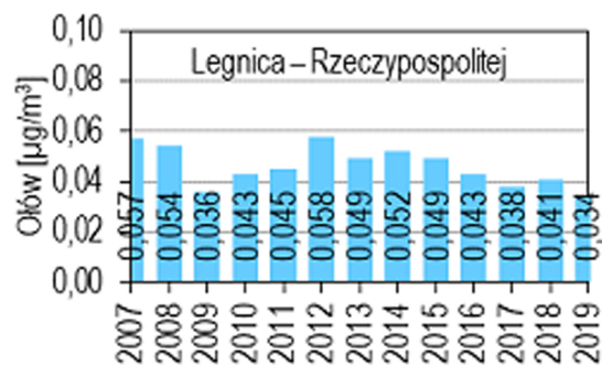
Wykres 14. Zmiany poziomu stężeń średniorocznych ołowiu, kadmu, niklu, arsenu w pyłe PM10 w wybranych stacjach województwa dolnośląskiego
