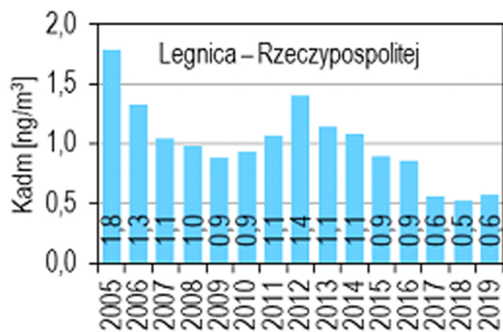
Wykres 14. Zmiany poziomu stężeń średniorocznych ołowiu, kadmu, niklu, arsenu w pyłe PM10 w wybranych stacjach województwa dolnośląskiego
